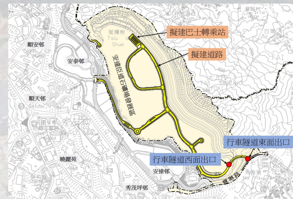
安達臣道發展區內的擬建交通網絡
